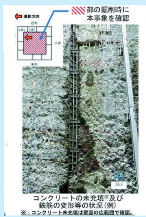
▲日本原電発表資料より「コンクリート未充填は壁面の広範囲で確認」とあります。
