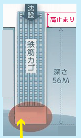
▲計画の深さまで基礎の鉄筋が届いていない。(告発者の情報より作図)
