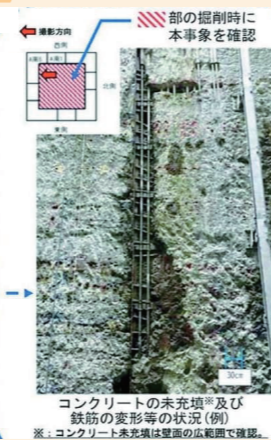
▲日本原電発表資料より「コンクリート未充填は壁面の広範囲で確認」とあります。
