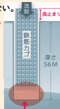
計画の深さまで基礎の鉄筋が届いていない。(告発者の情報より作図)
